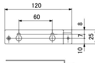
(壁掛け金具外形寸法)
